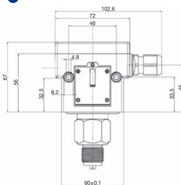
2 Gehäuse 300 (Klemmenanschluss)
