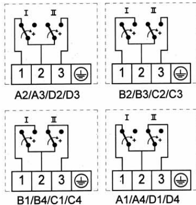
Abb. 15. Anschlußpläne ...-217
