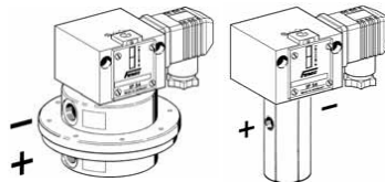
Abb. 4. Druckanschluß
