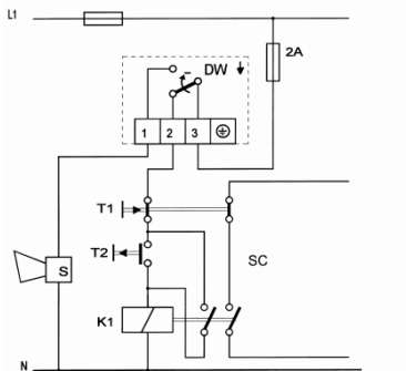
Abb. 7. Minimaldruckbegrenzung
