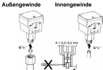
Abb. 3. Druckschalter
