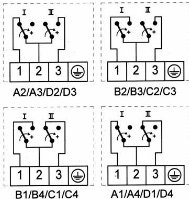
Abb. 15. Anschlußpläne ...-217
