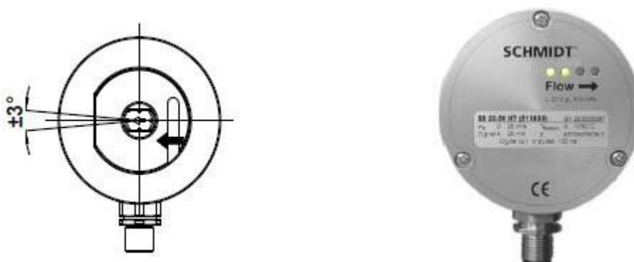
Abbildung 3-2 Anordnung Strömungsrichtungspfeile
